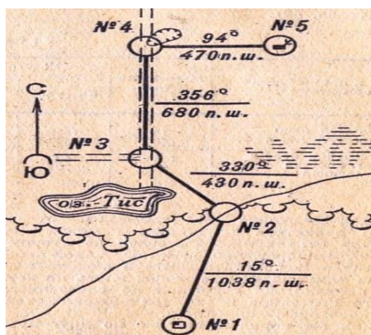
Рис. 5.7 Схема маршрута для движения по азимутам Таблица 5.2
